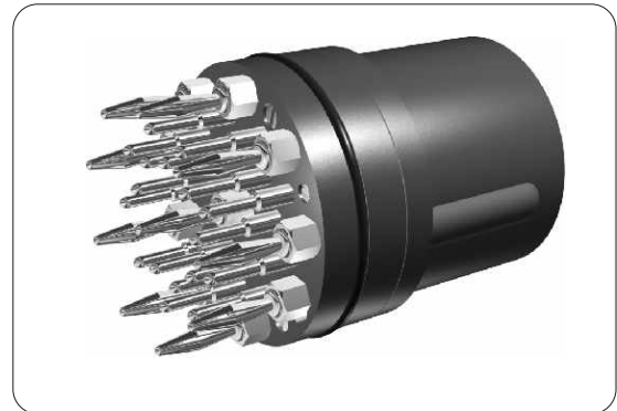
直式电缆28芯插针插头 Straight Cable 28 Pins Plug
